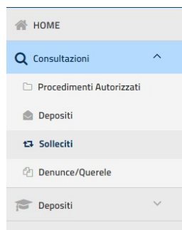
Figura 5 - Menù PDP
