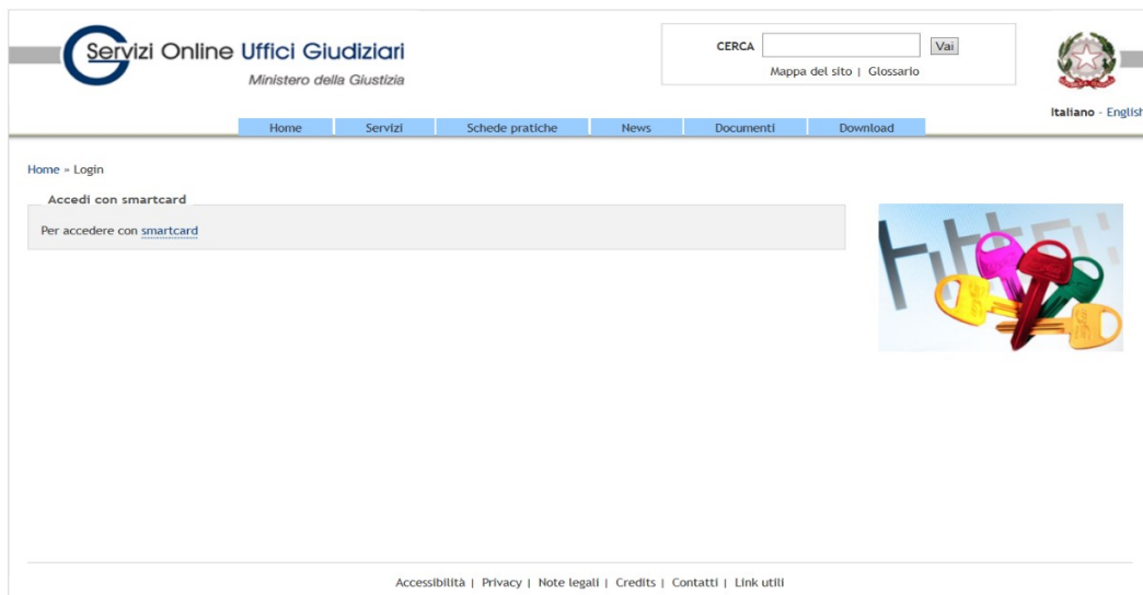
Figura 1 - Accesso PST
